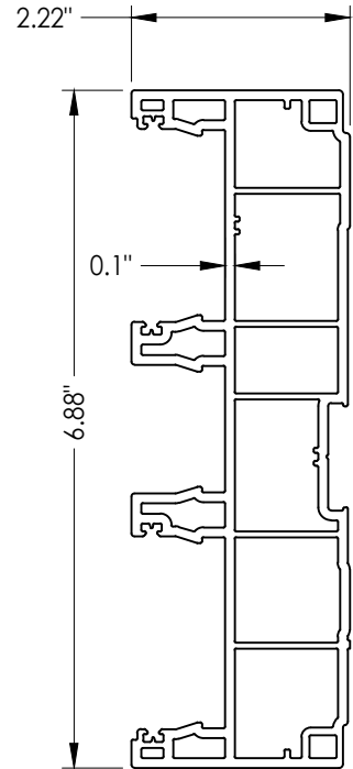
34 FRAME JAMB
