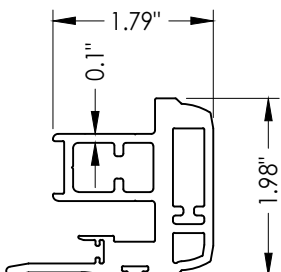
52 INTERLOCK
